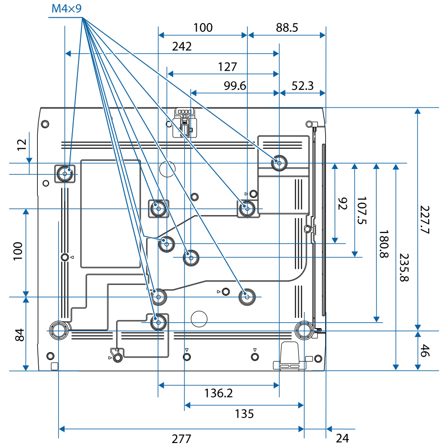
2 從投影鏡頭中心至天花板吊架固定點的距離
