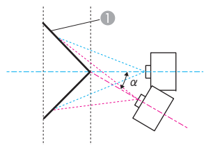
顶部视图
