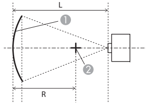
Üstten görünüm
