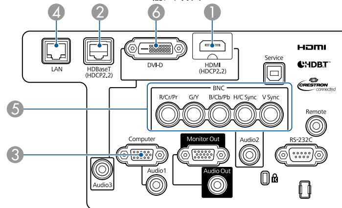
输入端口
