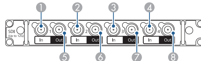
SDI 인터페이스 보드(ELPIF02)
