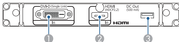
HDMI/DVI-D 인터페이스 보드(ELPIF01)
