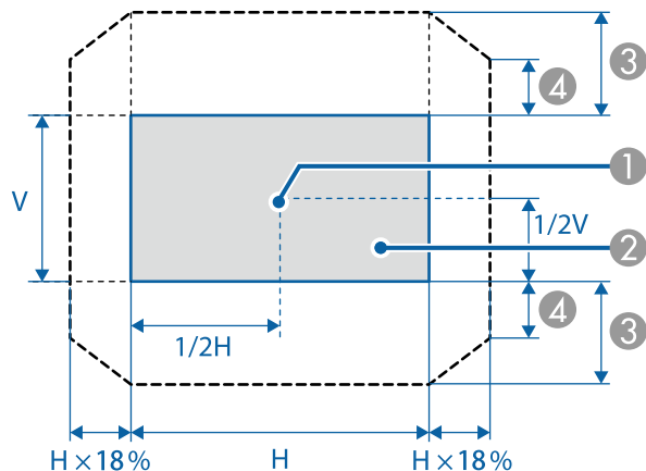
ELPLU04/ELPLW06/ELPLW08/ELPLM09/ELPLM10/ELPLM11/ELPLM15/ ELPLL08使用時
