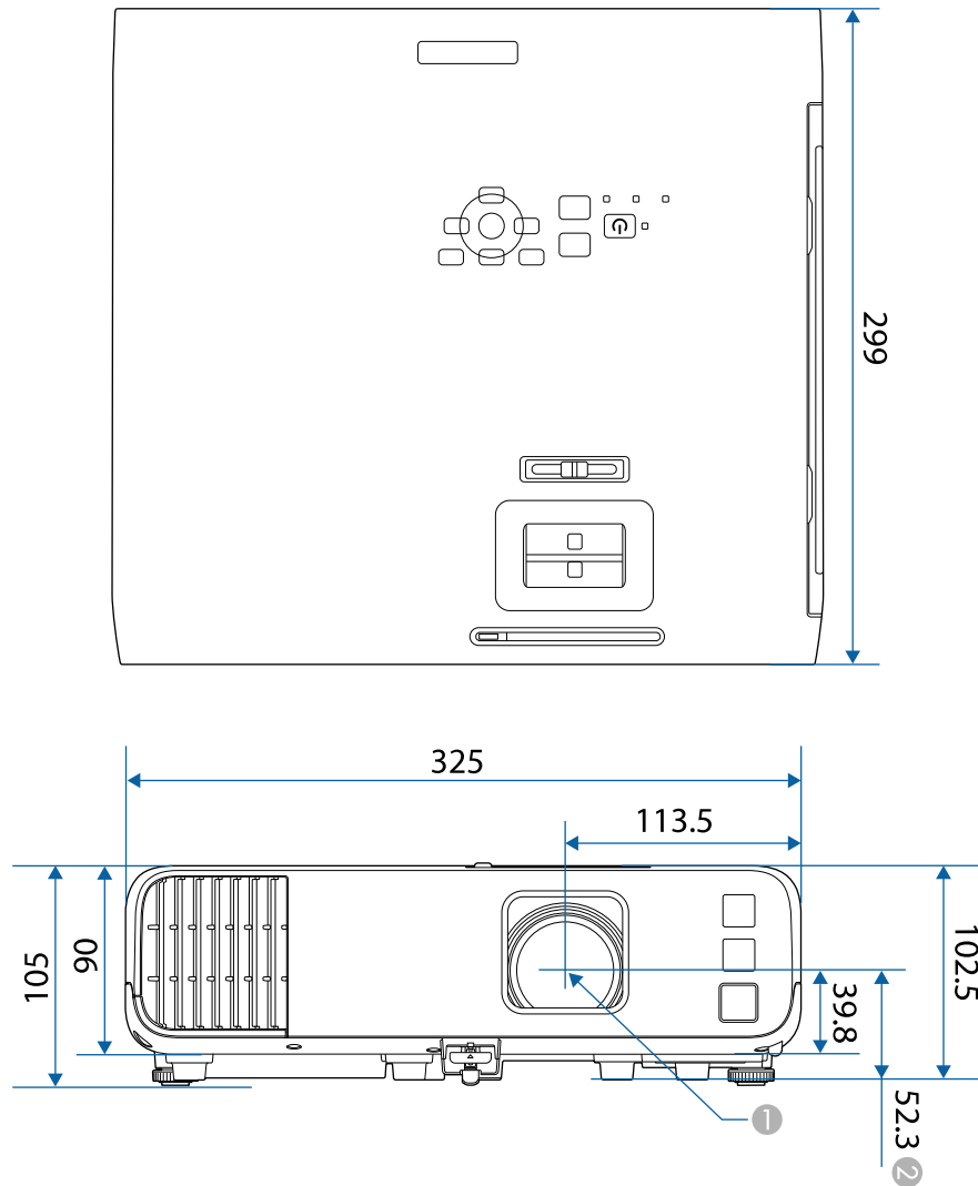
① 투사 렌즈 중앙
