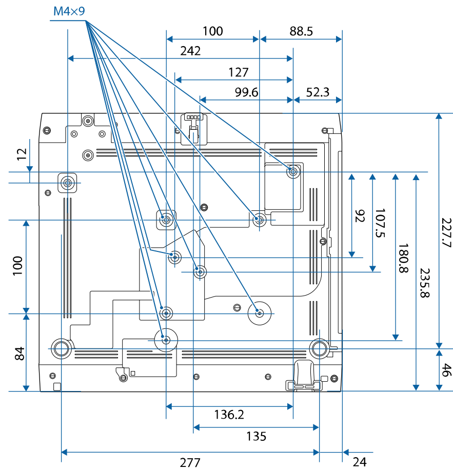
2 從投影鏡頭中心至天花板吊架固定點的距離
