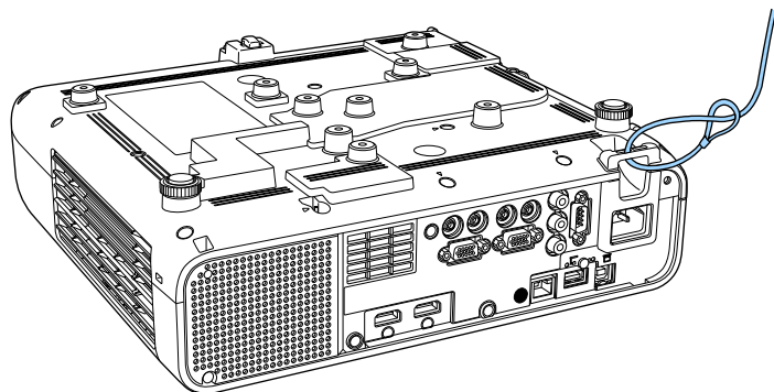
安装电缆盖时 (EB-L265F)
