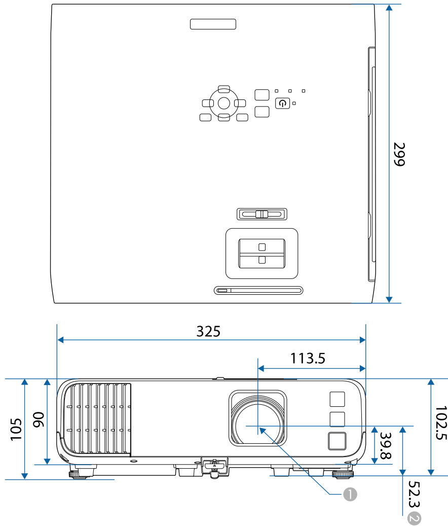
① 投影镜头中心
