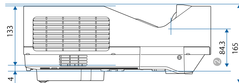
❷ 投写レンズの中心から天吊り金具固定部まで
