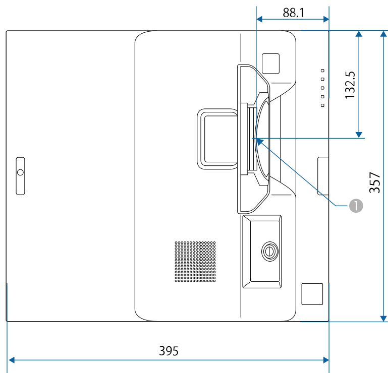
❶ 投写レンズの中心
