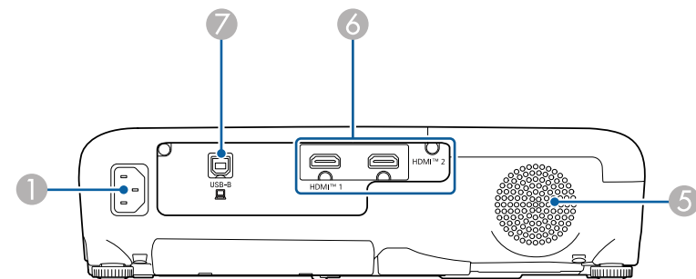
EB-W53/EB-E12/EB-EA12
